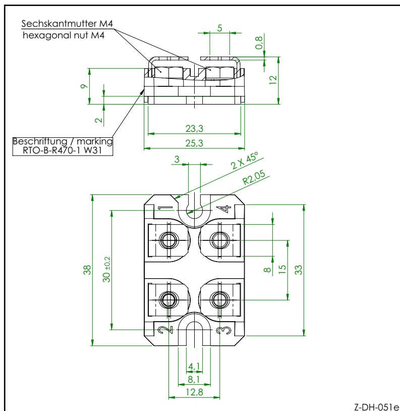
Abmessungen (mm) / dimensions (mm)
