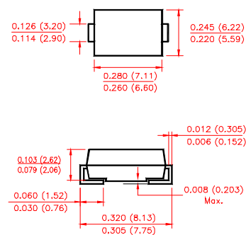
DO-214AB(SMC)
