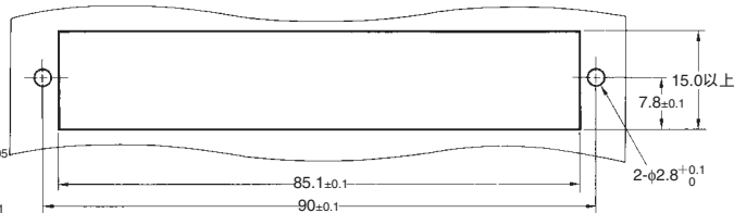
面板加工尺寸
