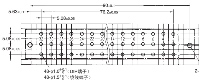
印刷基板加工尺寸 （BOTTOM VIEW）
