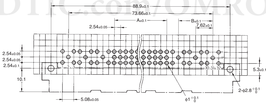
尺寸表
