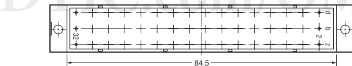
印刷基板加工尺寸 （BOTTOM VIEW）
