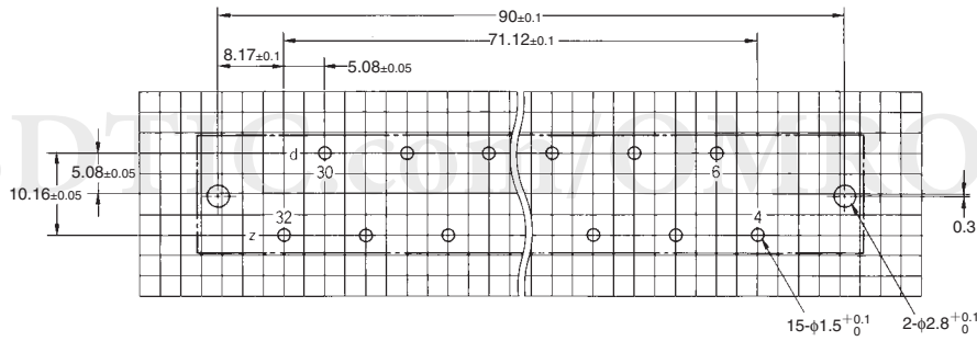
印刷基板加工尺寸 （BOTTOM VIEW）
