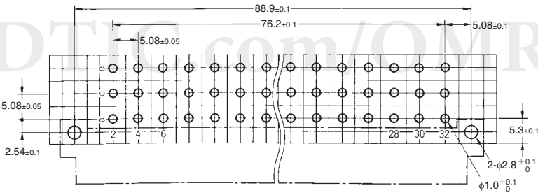
印刷基板加工尺寸 （BOTTOM VIEW）
