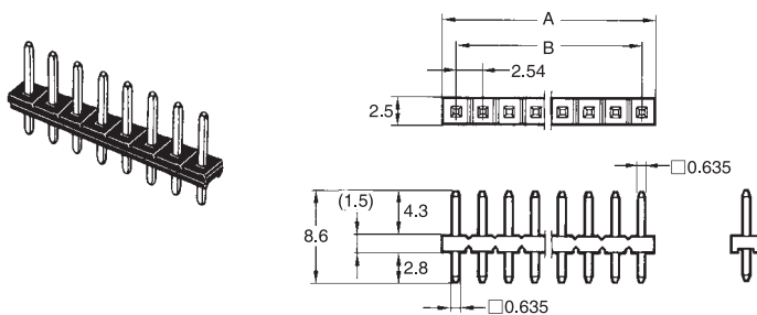
1列型/XJ8B-□□11
