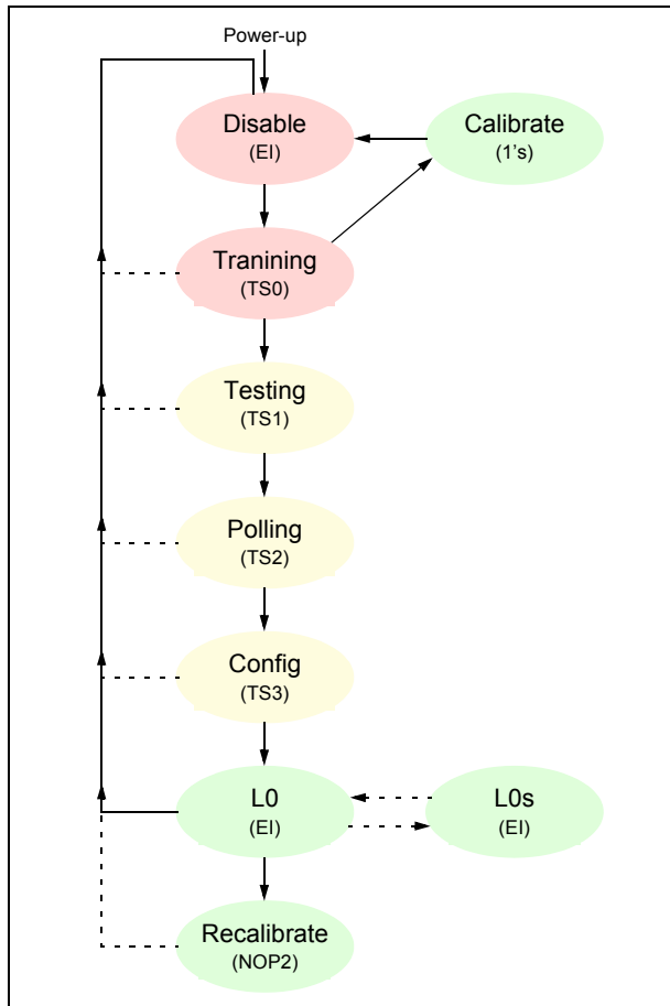
Figure13 : AMB Initialization Flow Diagram
