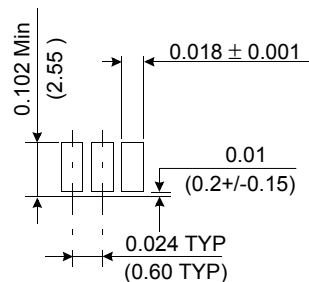
Detail Y
