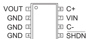
SC70JW-8
