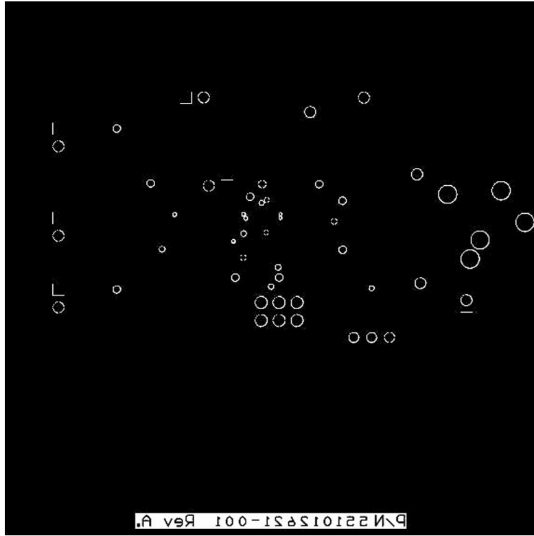
Bottom Layer
