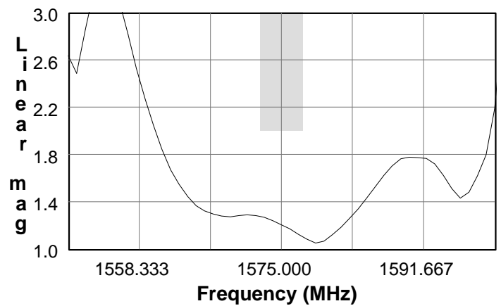
S11 VSWR
