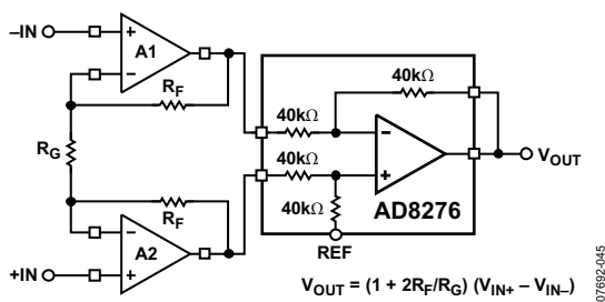
图52. 低功耗、精密仪表放大器
