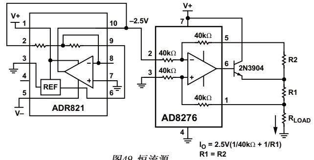
图49. 恒流源
