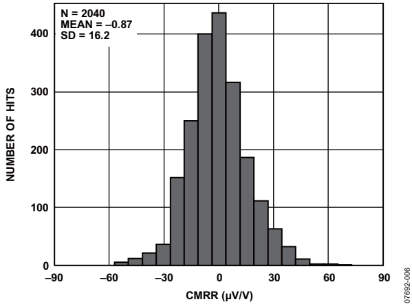
图8. 典型共模抑制分布图
