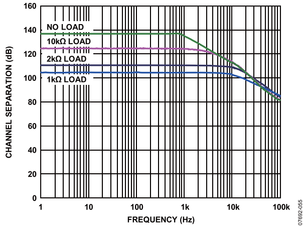
图37. 通道隔离
