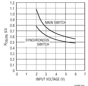
R_{DS(ON)} 与输入电压的关系曲线
