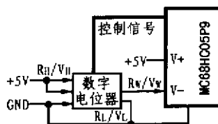
图 4 量程自动转换参考电源控制电路
