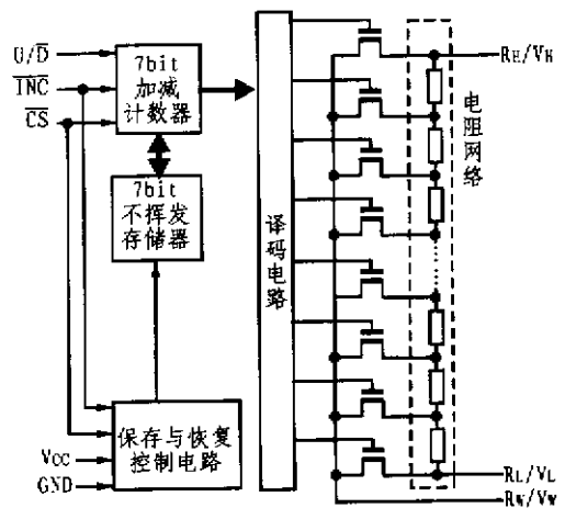
图 1 X9C 系列数字电位器的内部结构
